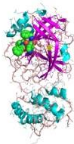
Estructura del complejo formado por SARS coronavirus proteasa y el alfa-cetoamida(S)-N-bencil-3-((S)-2-cinnamamido-3-fenilpropanamido)-2-oxo-4-((S)-2-oxopirrolidin-3-il) butanamida .
