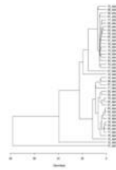
Análisis de agrupamientos para la similitud molecular de diferentes moléculas, usando los campos escalares de deformación de la densidad y potencial electrostático.
